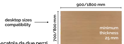
spot-gamba pieghevole d.35 h.700 per piano da 700 con accessori-scatoia da due pezzi spot-leg folding d.35 h.700 to plan for 700 with accessories-two pieces box
